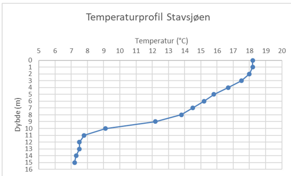
Figur 15: Temperaturprofil fra Stavsjøen den 19. august 2020.
